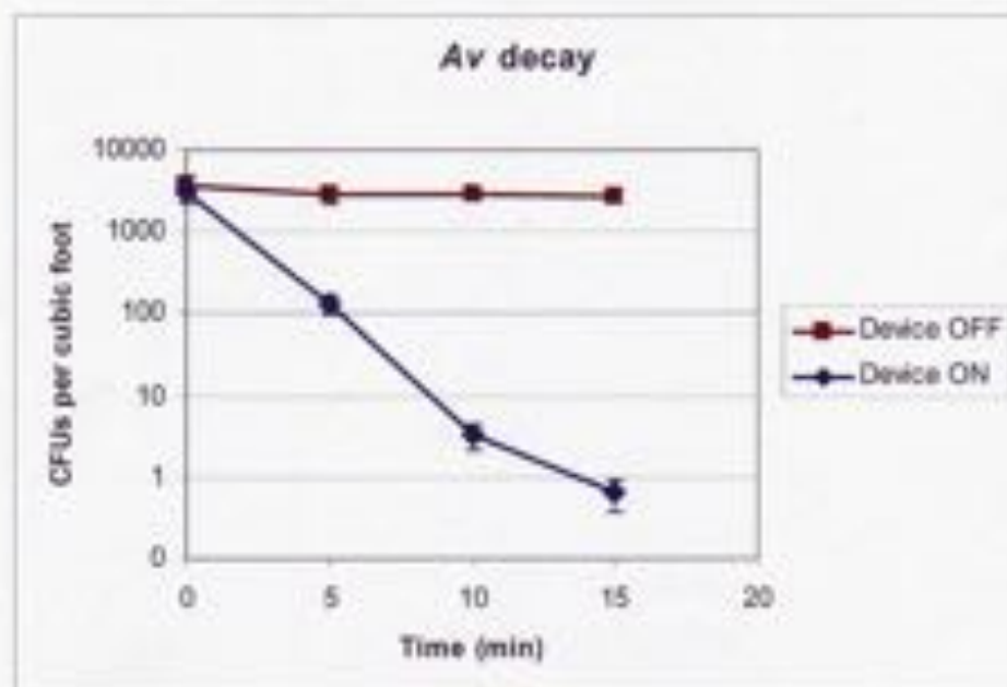
Figure 5. Decay curves for the Av fungal spores
